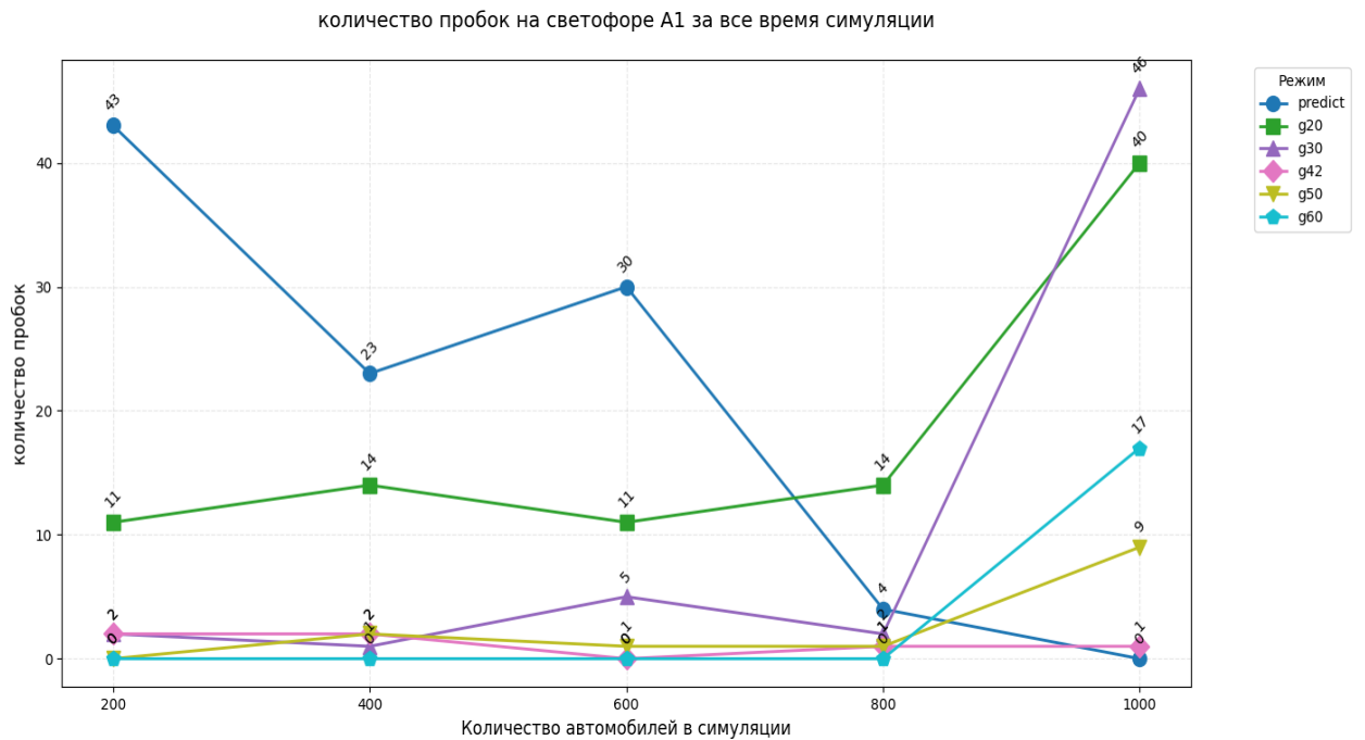
Рис 46. Количество пробок на светофоре A1 за все время симуляции.
