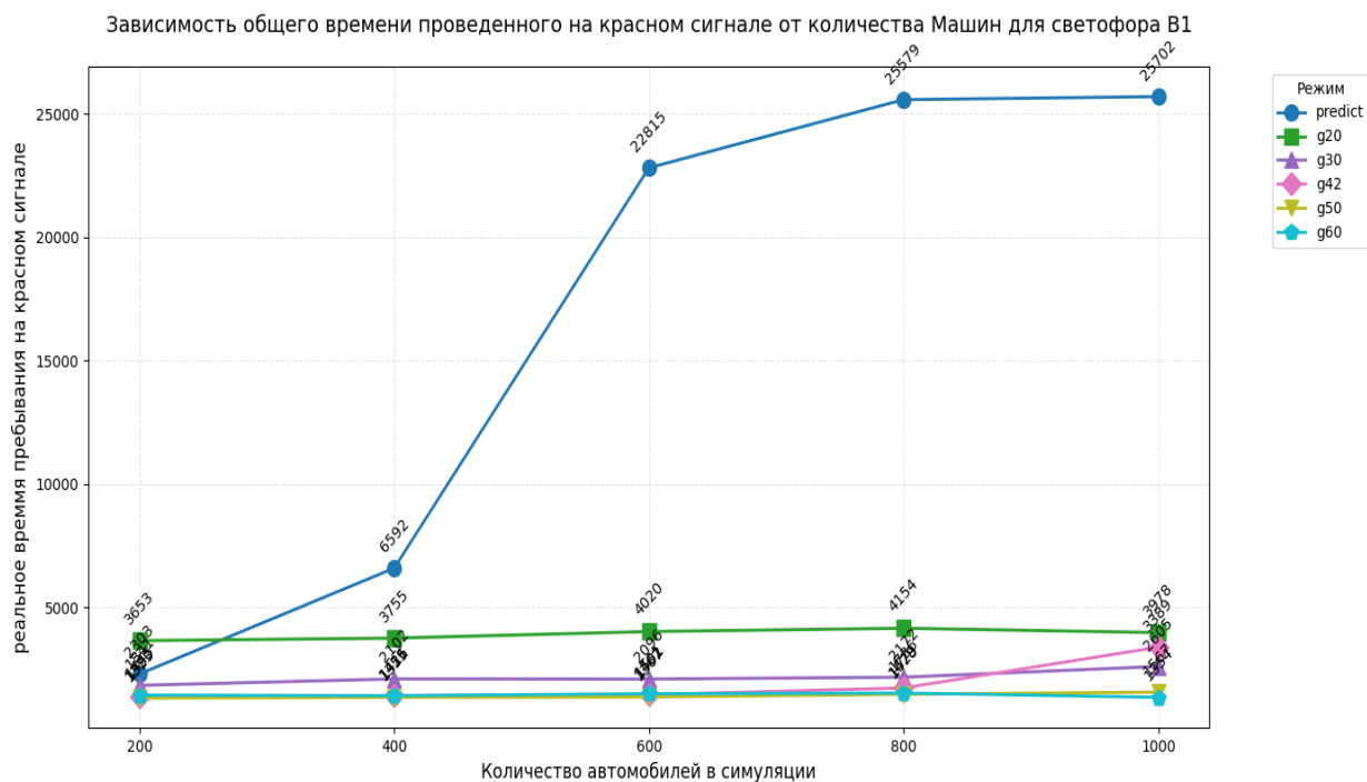
Рис 41. Зависимость общего времени, проведенного на красном сигнале от количества машин в симуляции для светофора В1.
