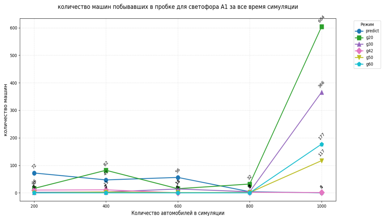
Рис 47. Количество машин, побывавших в пробке для светофора A1 за все время симуляции.
