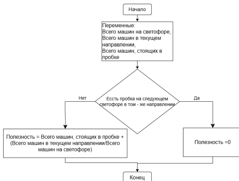
Рис 26. Алгоритм вычисления полезности переключения на зеленый сигнал для направления движения.
